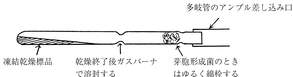
図30 凍結乾燥用アンプル
